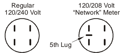
1-Ø Meter Base Lugs
